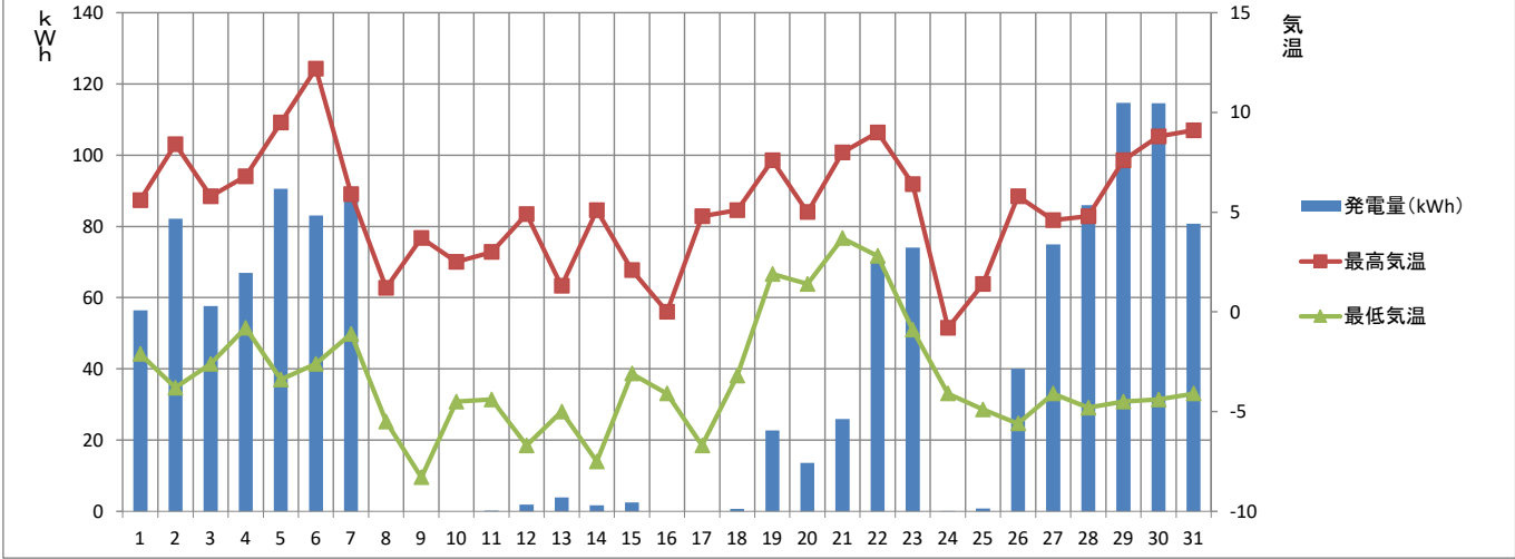
【2024年1月】 須坂市消防本部 発電量と気温の推移
