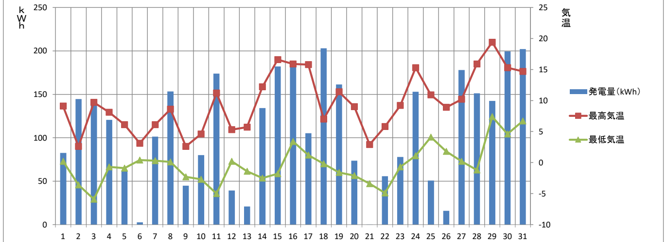
【2024年3月】 須坂市消防本部 発電量と気温の推移
