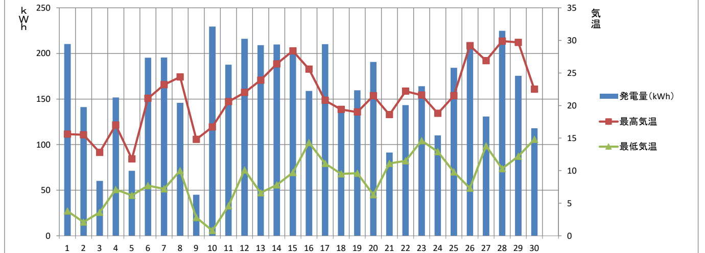
【2024年4月】 須坂市消防本部 発電量と気温の推移
