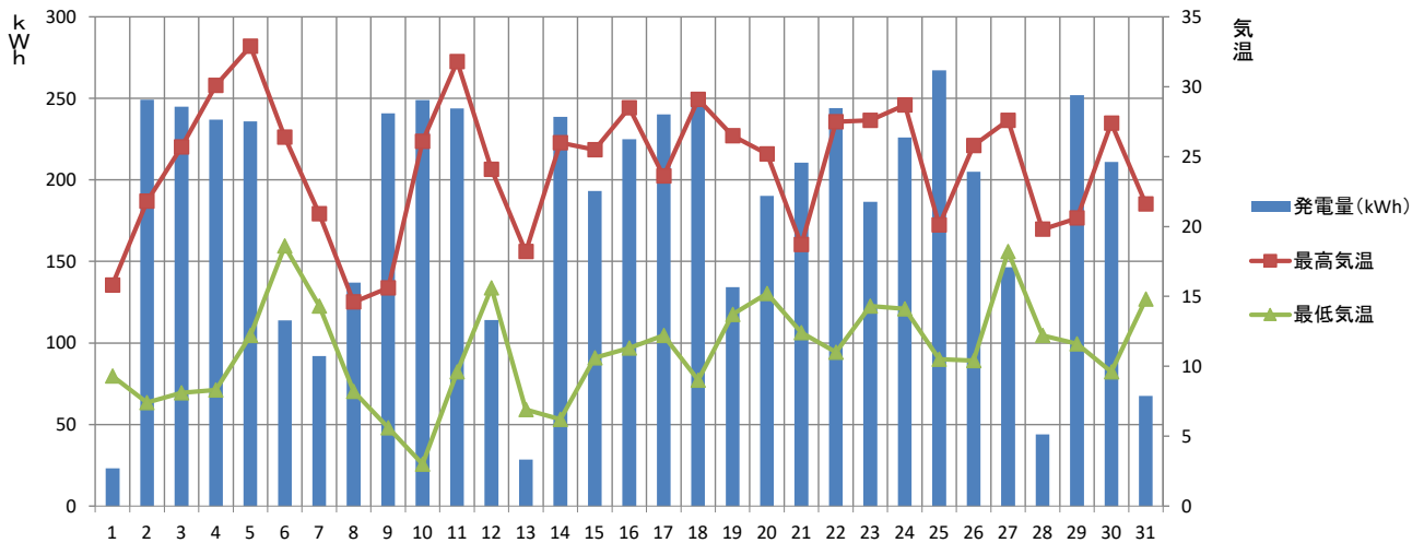
【2024年 5月】 須坂市消防本部 発電量と気温の推移
