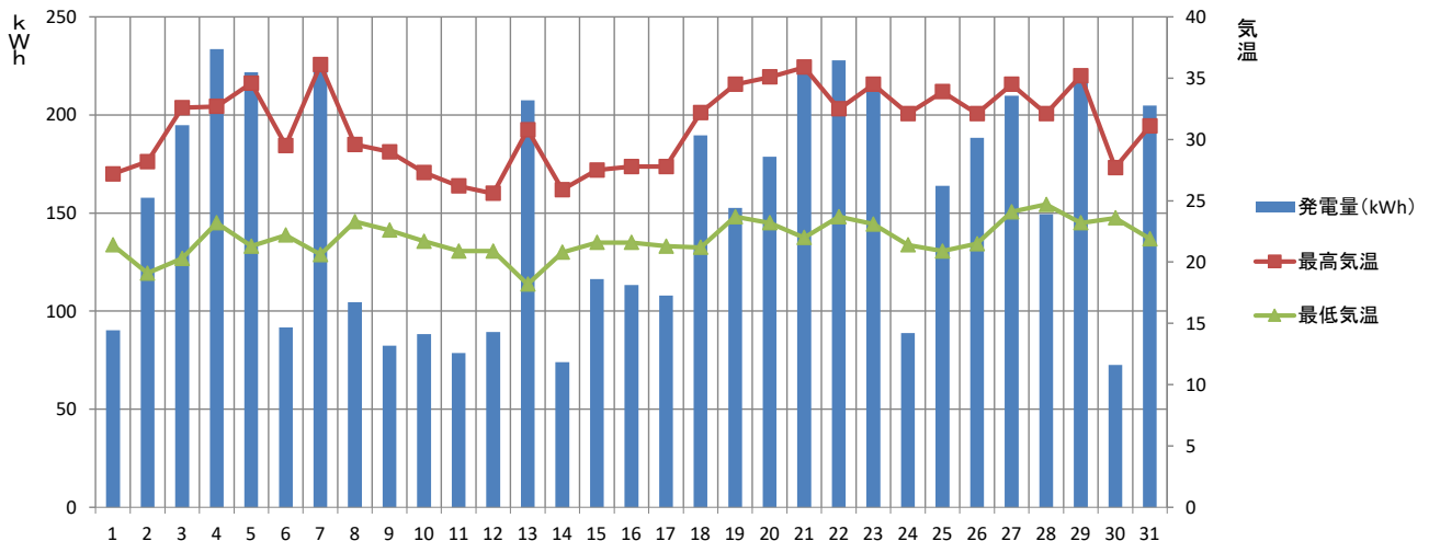
【2024年7月】 須坂市消防本部 発電量と気温の推移
