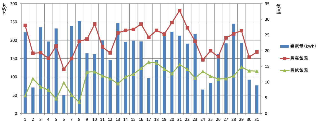
【2025年5月】 須坂市消防本部 発電量と気温の推移
