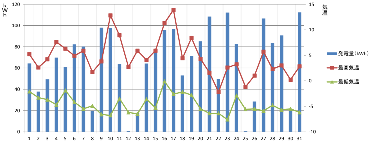
【2026年1月】 須坂市消防本部 発電量と気温の推移
