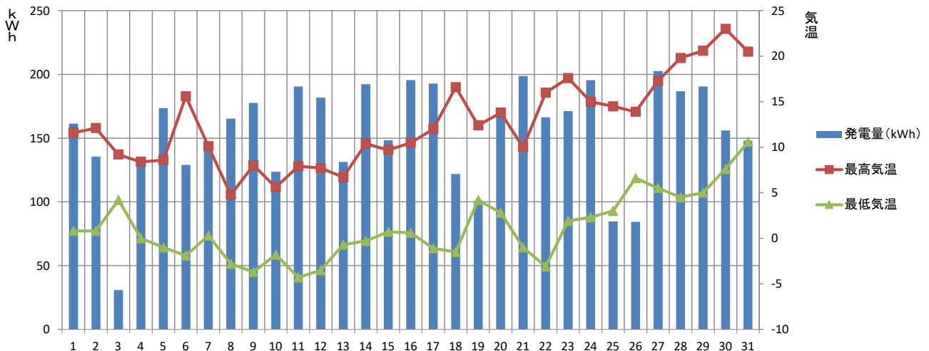
【2026年3月】 須坂市消防本部 発電量と気温の推移
