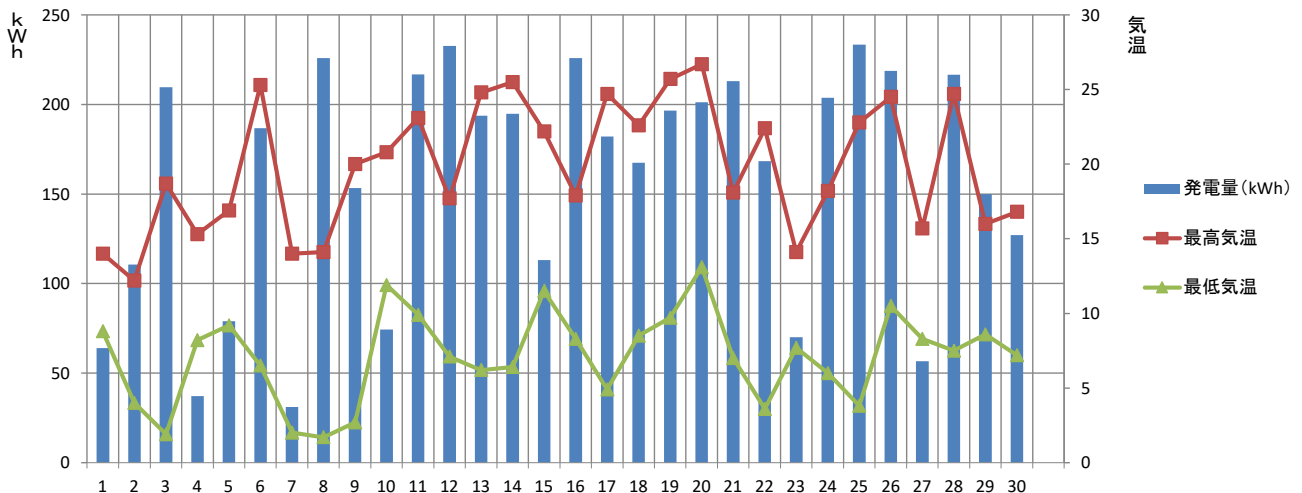
【2026年4月】 須坂市消防本部 発電量と気温の推移
